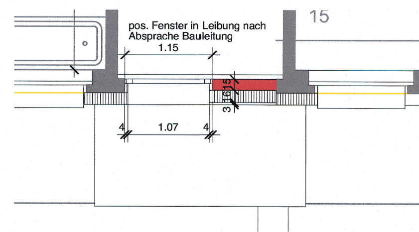
Grundriss Treppenfenster Obergeschosse
